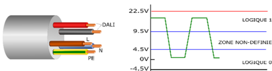
Figure 1 : Câblage typique et fluctuations en tension
