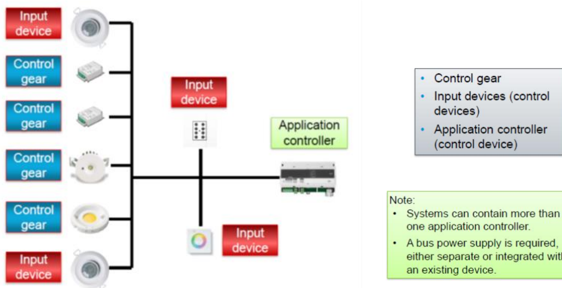
Figure 5 : Architecture d'un système DALI-2 (Source DiiA)
