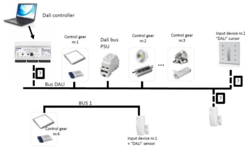
Figure 4 : Réseau avec deux bus DALI
