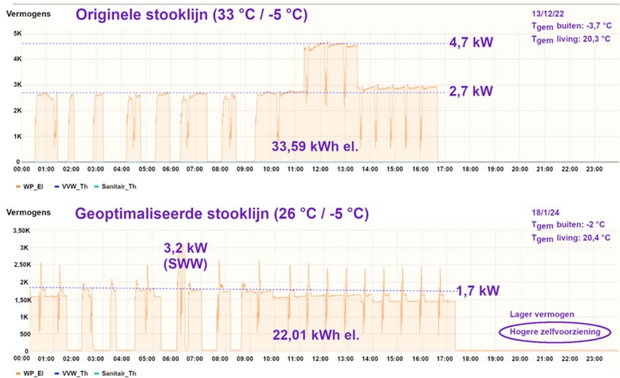
Grafiek 2: Het opgenomen elektrisch vermogen van de warmtepomp
