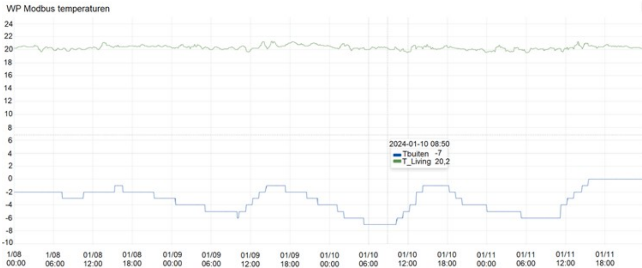
Grafiek 1: Binnentemperatuur bij vriestemperaturen bij een verlaagde afgiftemtemperatuur
