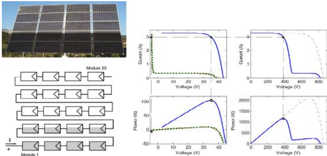
Figure 54 - Ombrage partiel sur une chaîne
