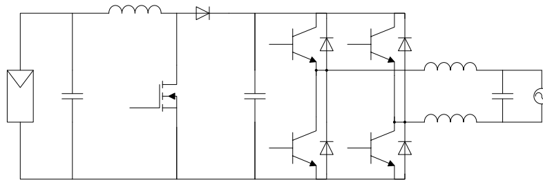
Figure 57 - Exemple d'onduleur sans transformateur
