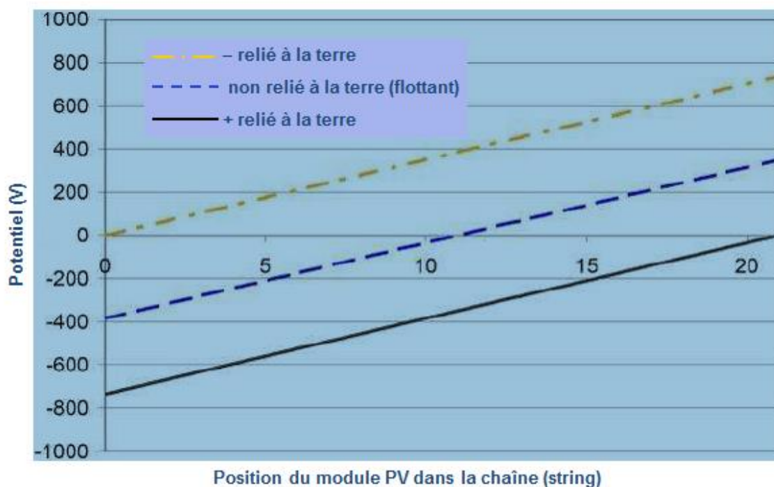
Figure 43 - Schémas de mise à la terre d'une installation PV de 750 V Source : [10]
