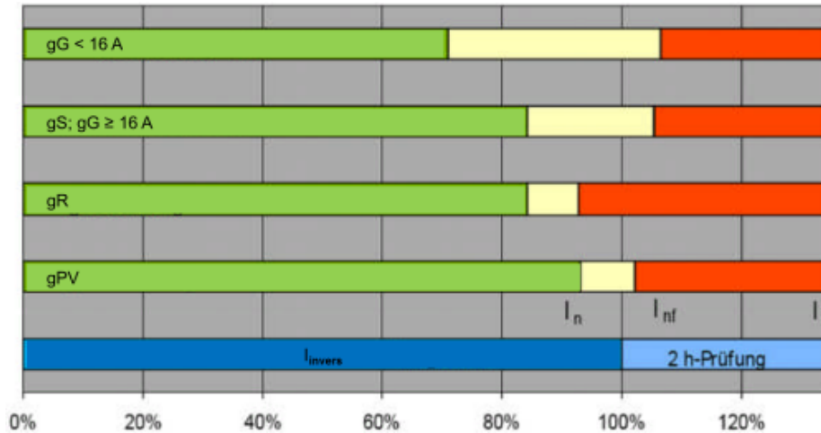
Figure 63 - Plage de fonctionnement de différents types de coupe-circuits à fusible avec I_f = 1,35 \times I_{invers\ mod}
