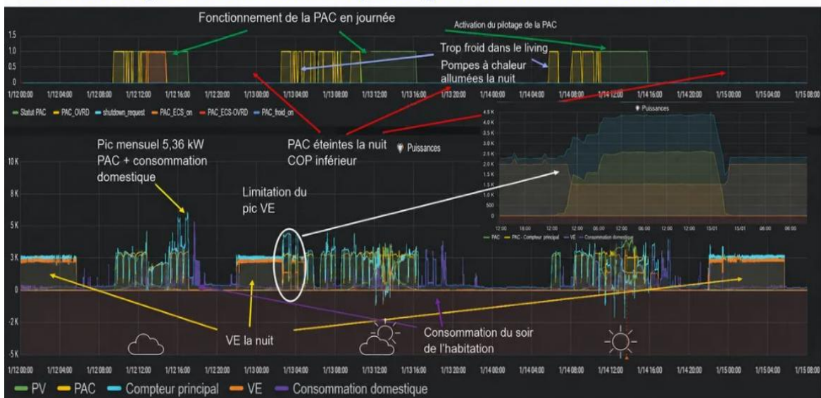
Figure 4: Pilotage via l'EMS de la pompe à chaleur et du véhicule électrique
