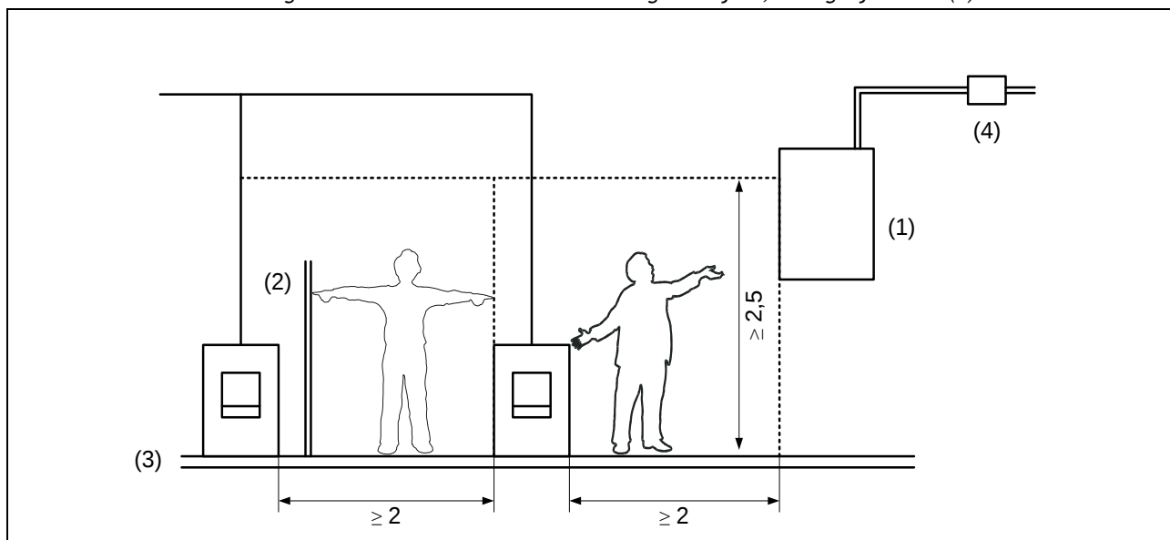
Figuur 4.2. Bescherming die de gelijktijdige aanraking van delen die op potentialen kunnen gebracht worden waarvan het verschil gevaarlijk is, onmogelijk maakt (2)
