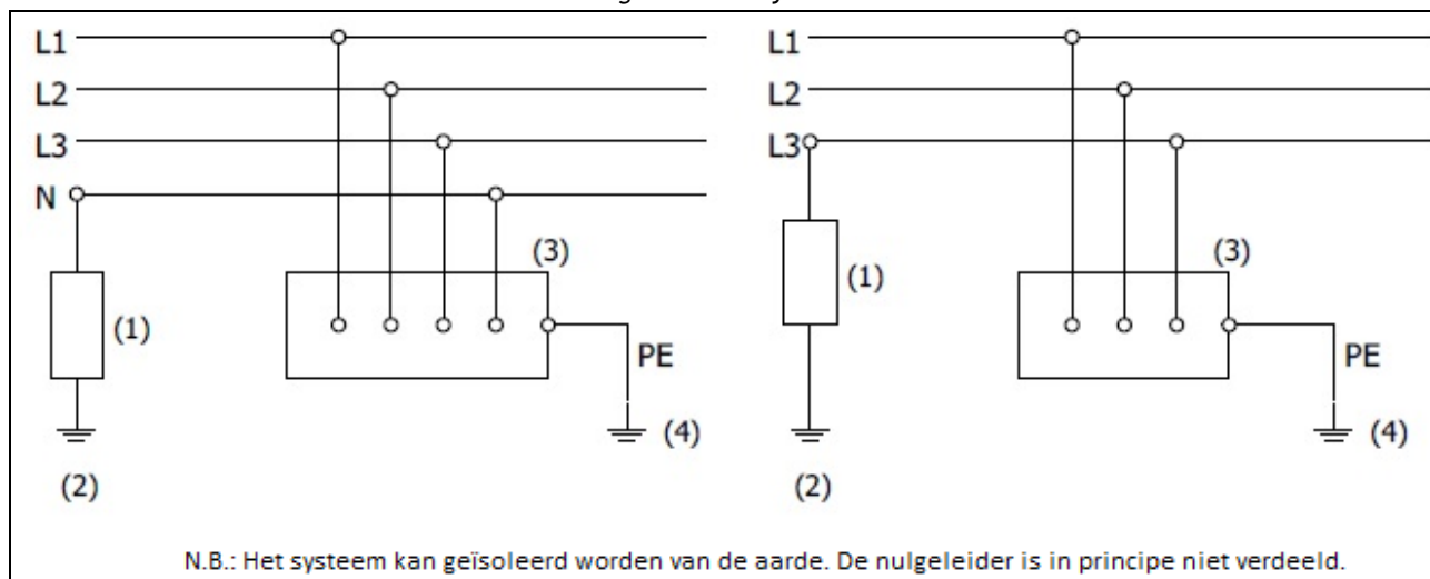
Figuur 2.5. IT-systeem
