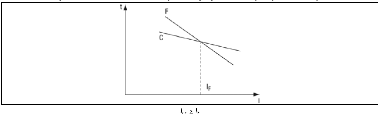
Figuur 5.29. Keuze van de beschermingsinrichting tegen kortsluitingen bij smeltzekeringen
