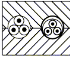
Figuur 5.20. Plaatsingswijzen van elektrische leidingen – Geprefabriceerde blokken
