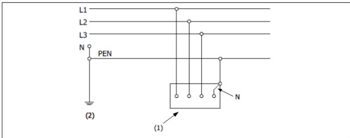
Figuur 2.2. TN-C-systeem
