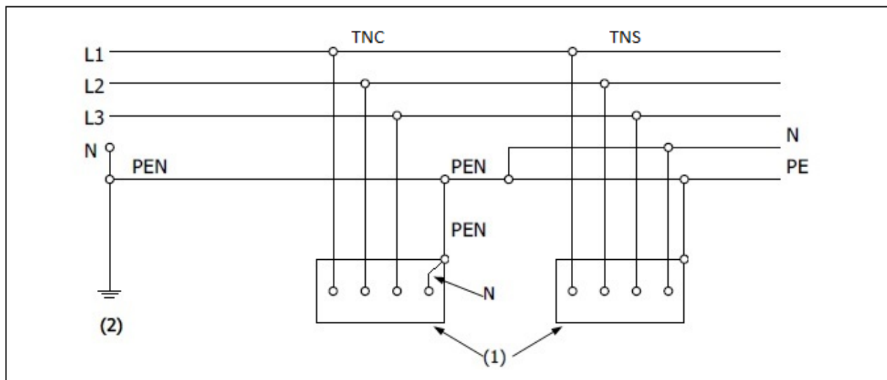
Figuur 2.3. TN-C-S-systeem
