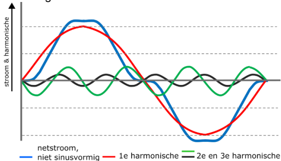
Fig.3: niet sinusvormige netstroom
