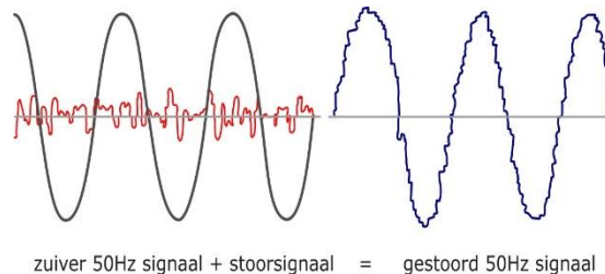
Fig.4: storing op de 50Hz netspanning
