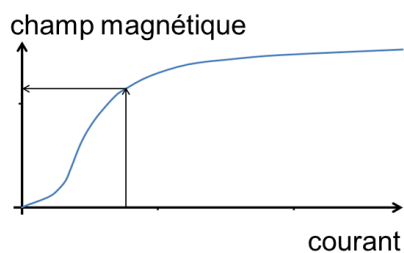
Figure 7 : relation entre le courant qui circule à travers le noyau magnétique et le champ magnétique créé
