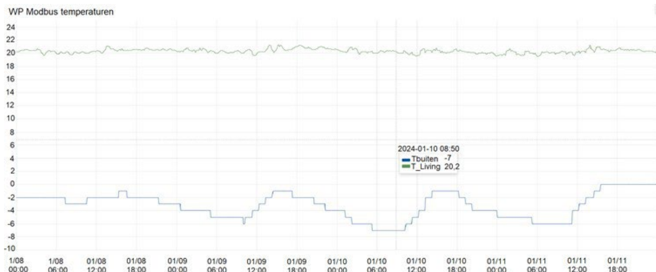
Grafiek 1: Binnentemperaturen bij vriestemperaturen bij een verlaagde afgiftetempera-tuur
