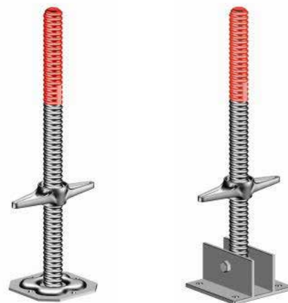
Figuur 23: Vaste en kantelbare voetspindel
