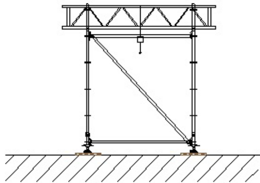
Figuur 13: Takelsteiger
