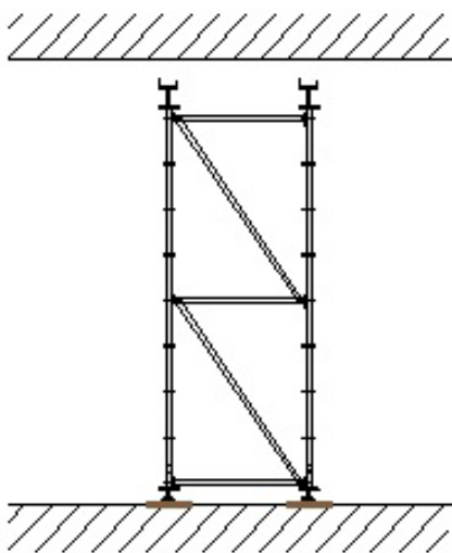
Figuur 14: Ondersteuning
