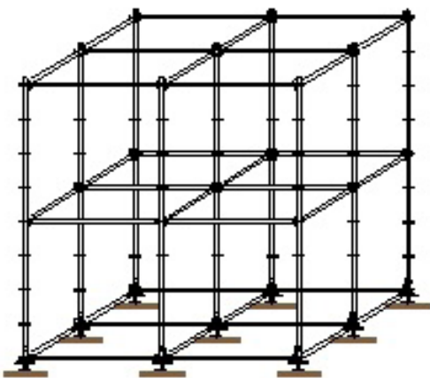
Figuur 7: Volumesteiger
