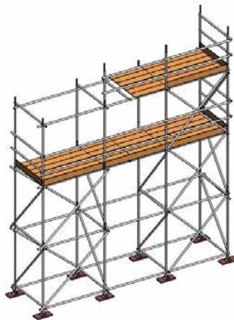
Figuur 3: Traditionele steiger
