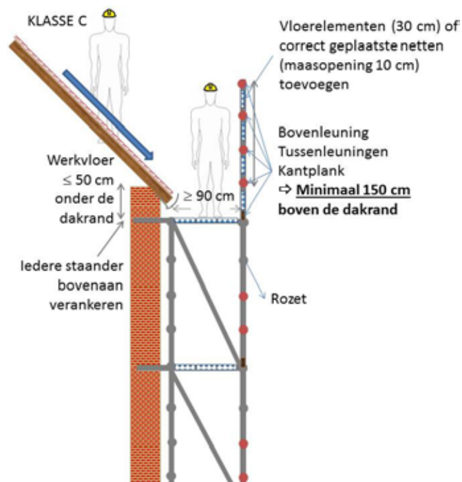
Figuur 25: Eisen leuning
