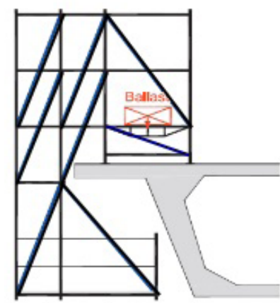
Figuur 29a: Ballast op 1 plaats
