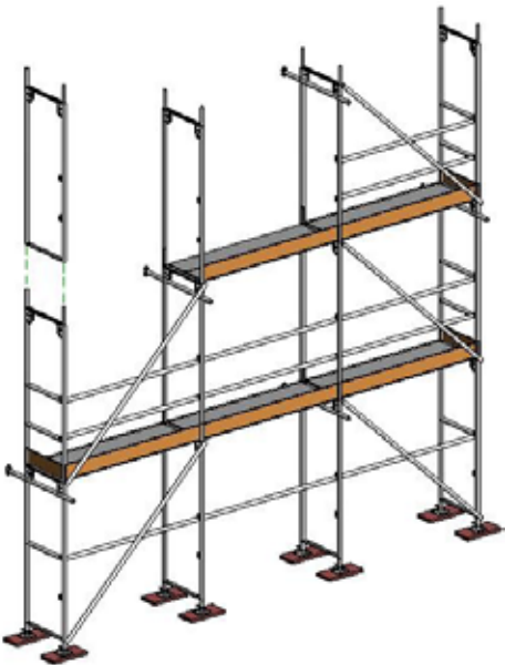
Figuur 2: Framesteiger
