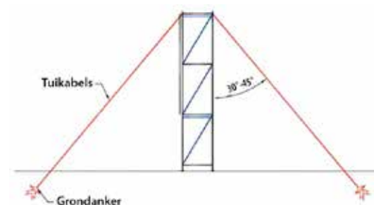
Figuur 30: Tuien
