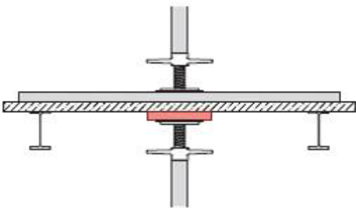
Figuur 21: doorstempeling vermijden
