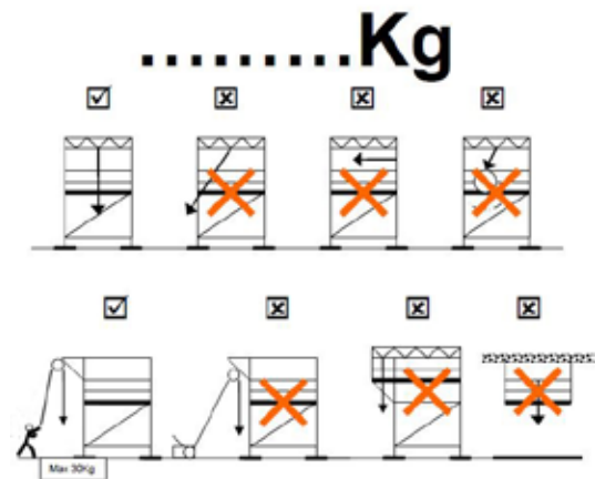
Figuur 34: Voorbeeld van een takellabel
