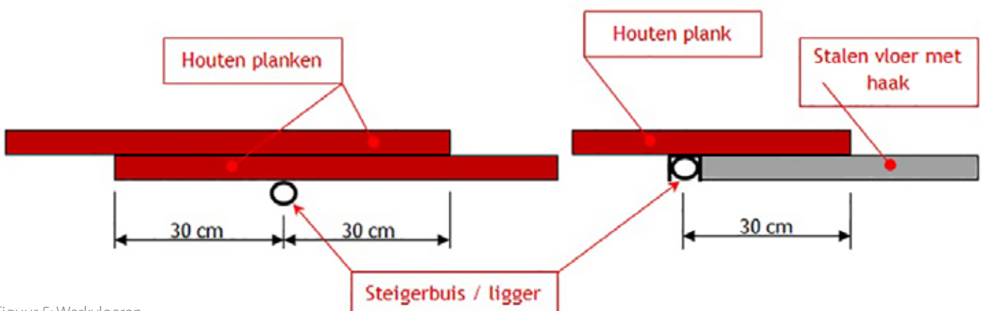
Figuur 5: Werkvloeren
