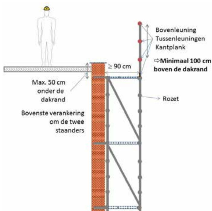
Figuur 24: Eisen opvangvloer
